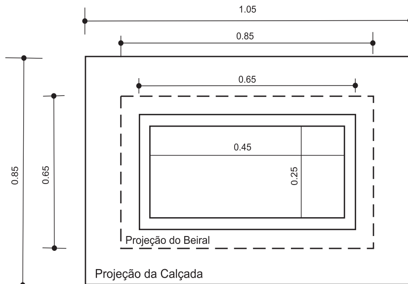
Planta Baixa Desenho s/Escala
